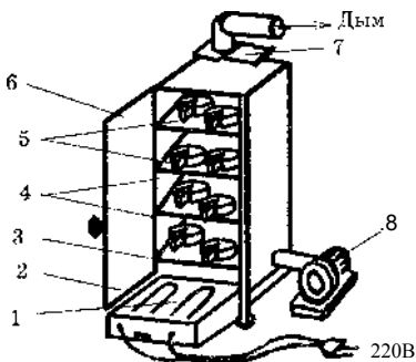
Рис. 3. Электрокопильный шкаф:
